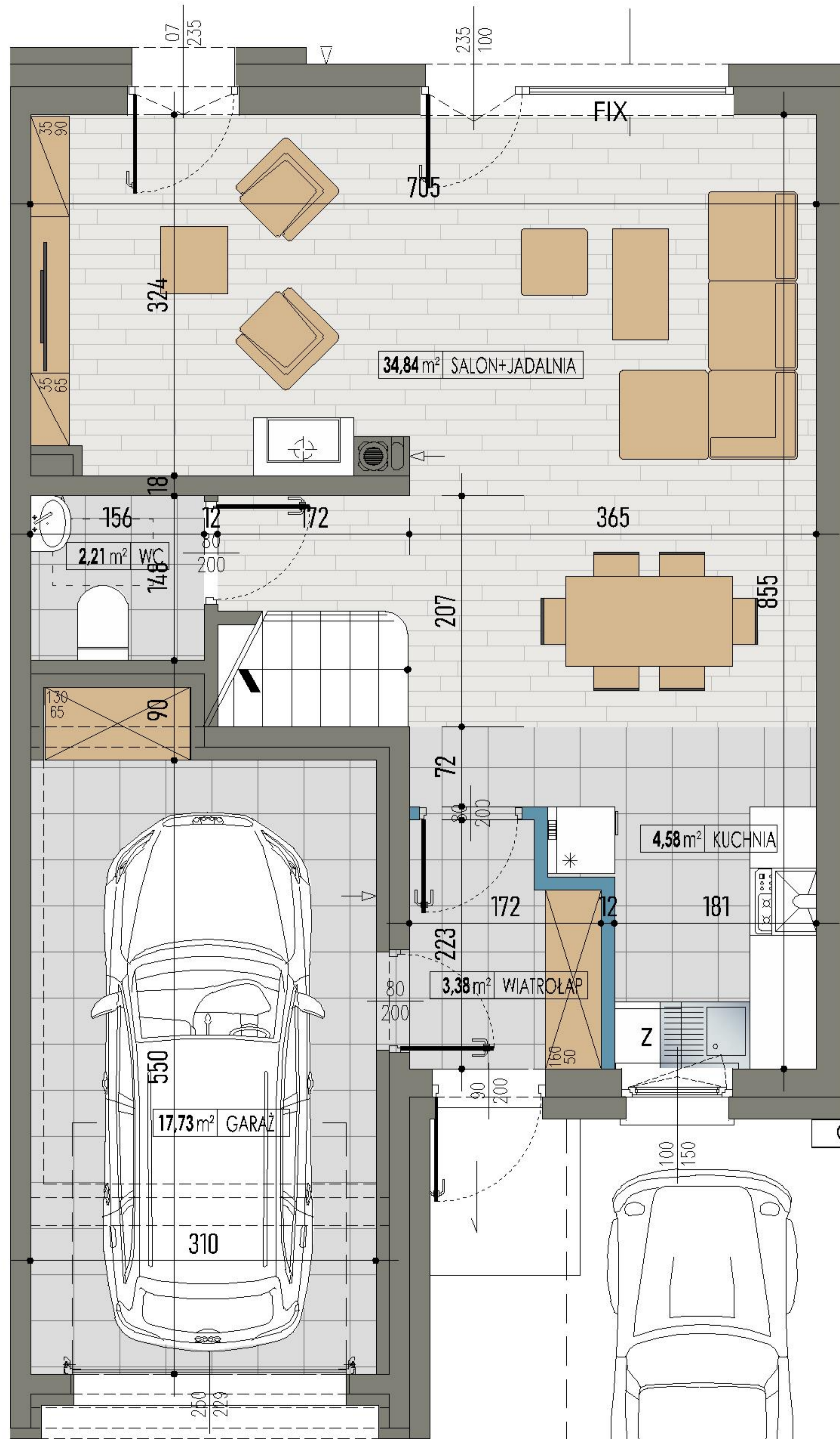
RZUT PARTERU
