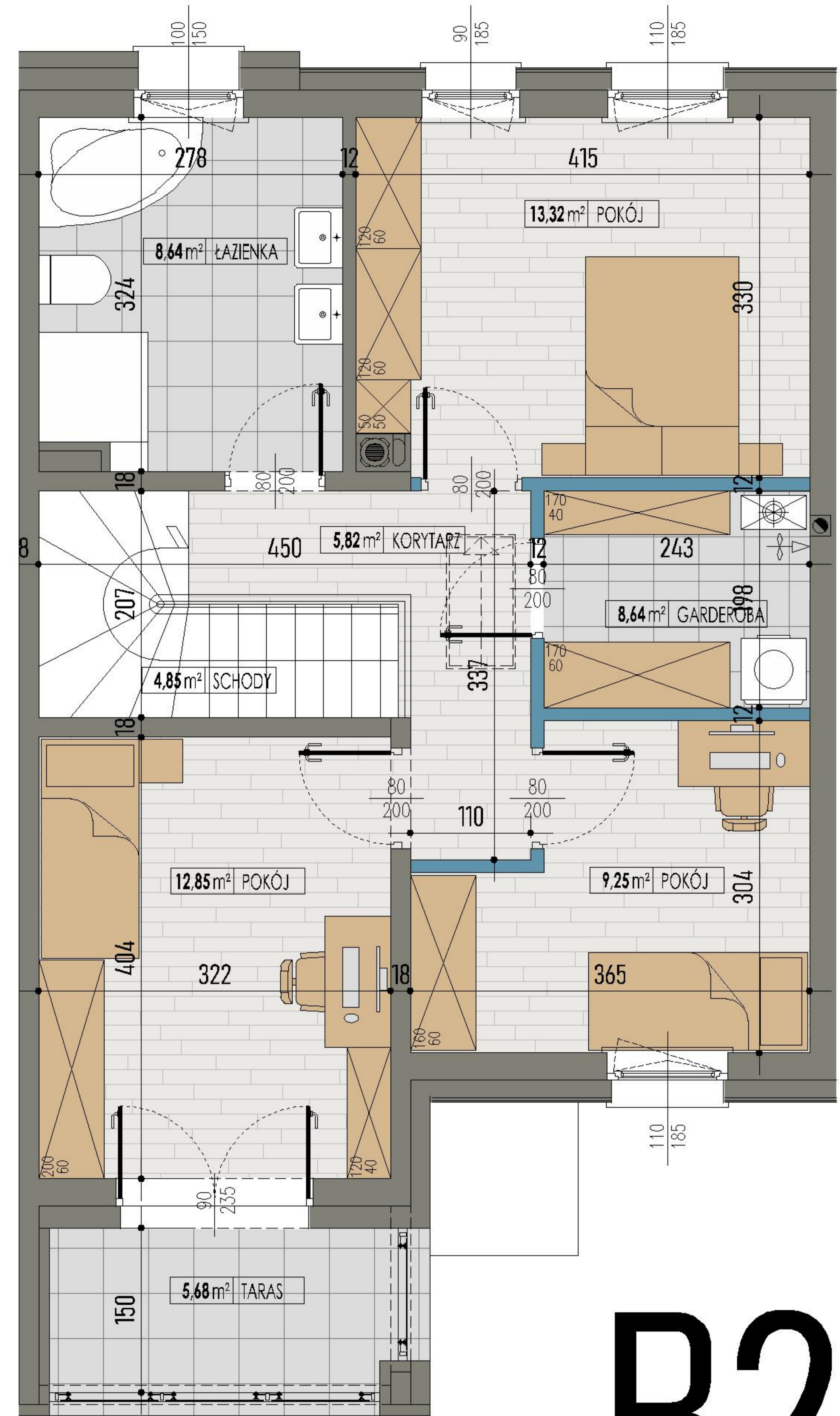
RZUT PIĘTRA
