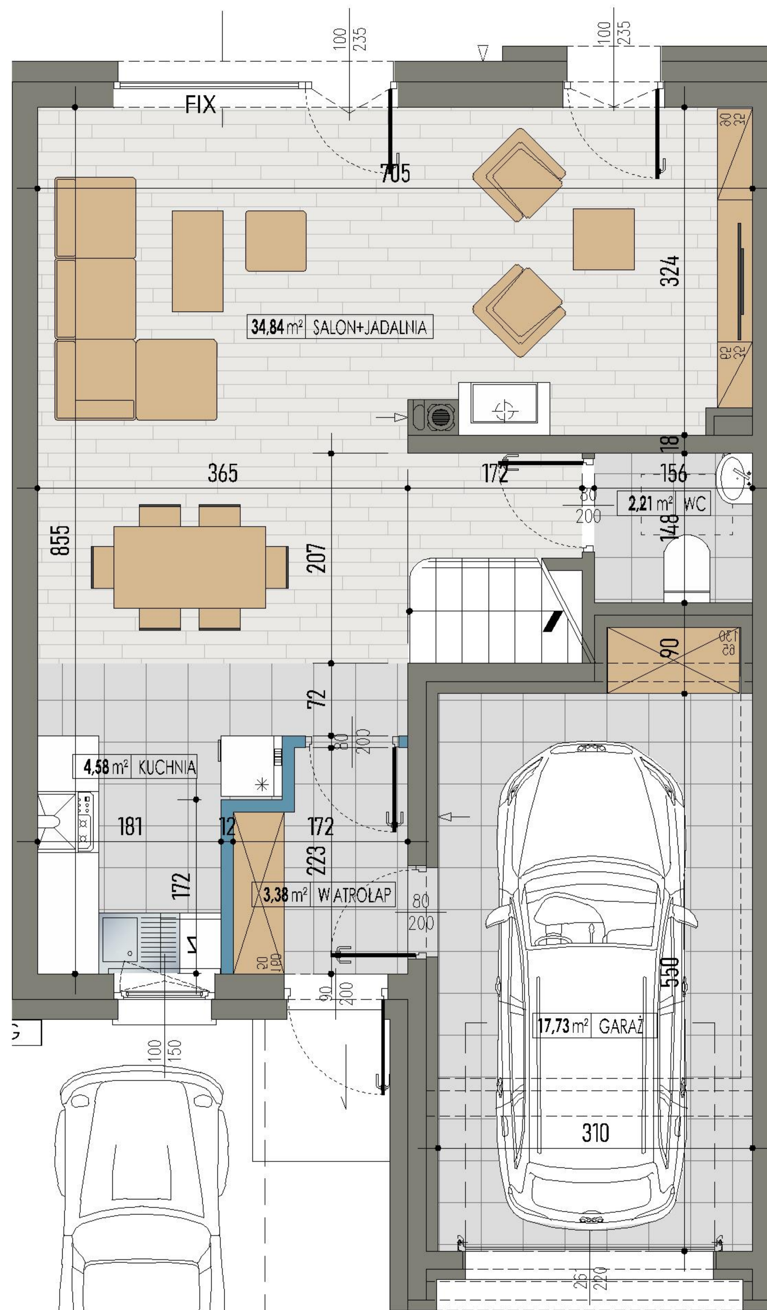
RZUT PARTERU
