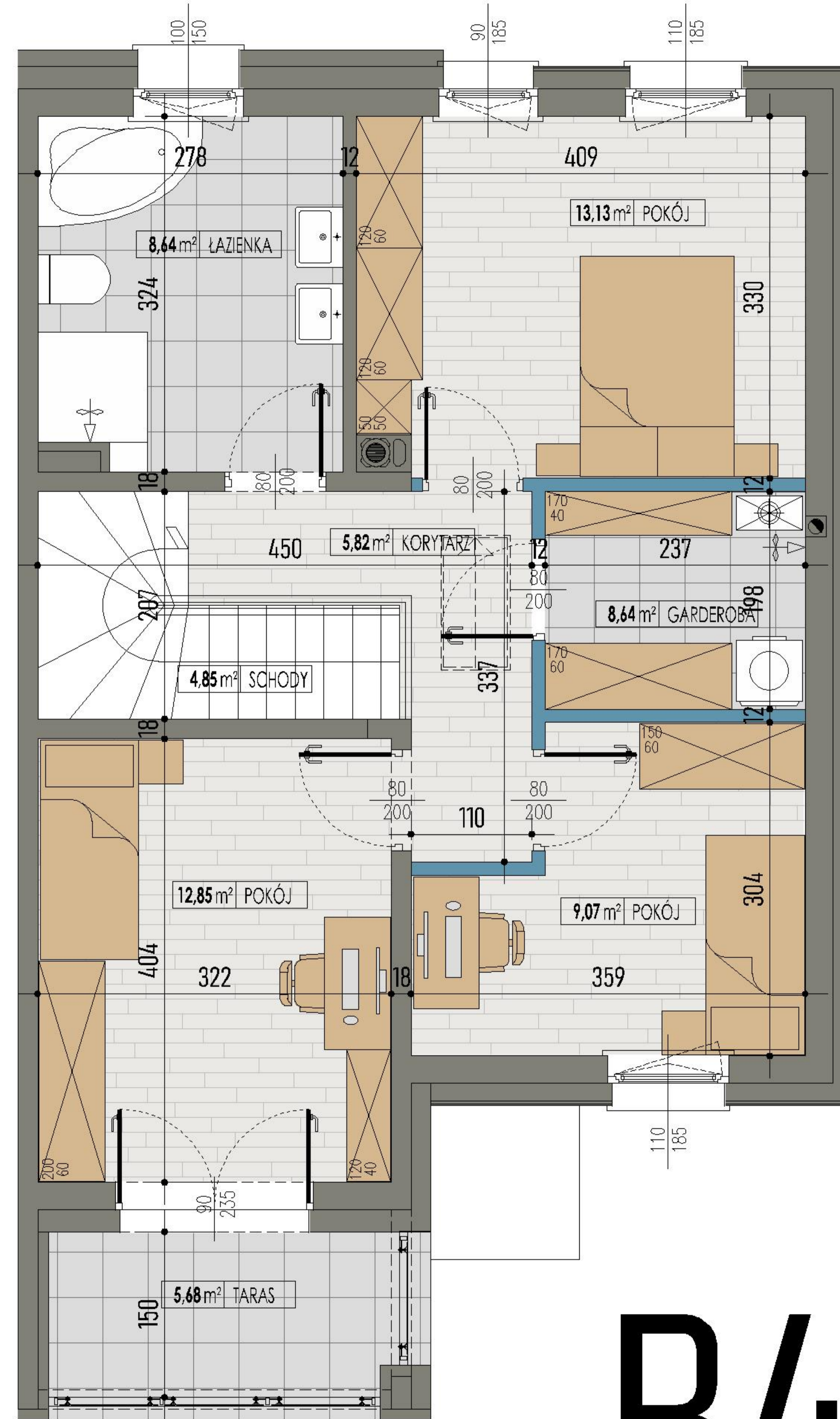
RZUT PIĘTRA
