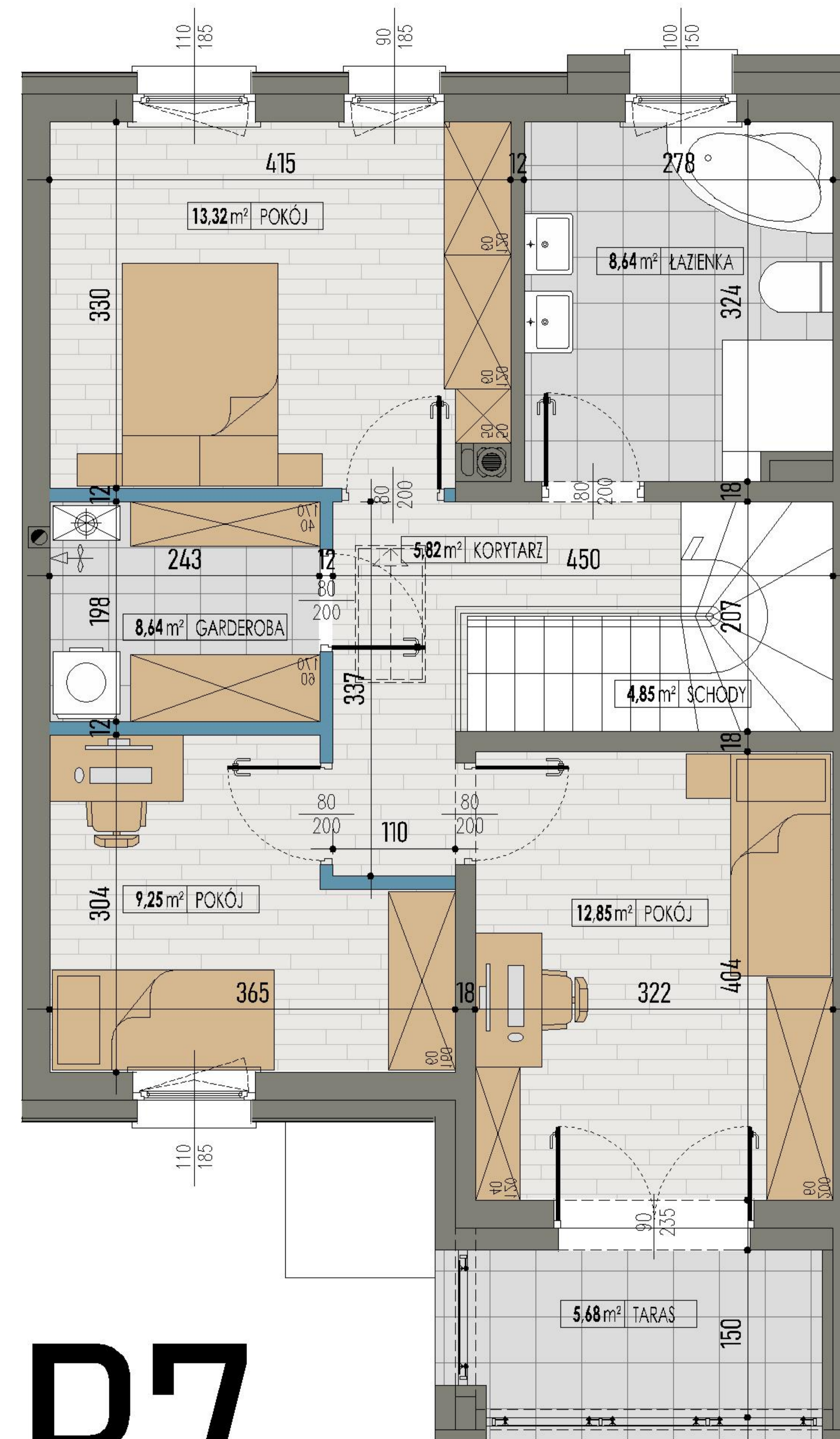
RZUT PIĘTRA
