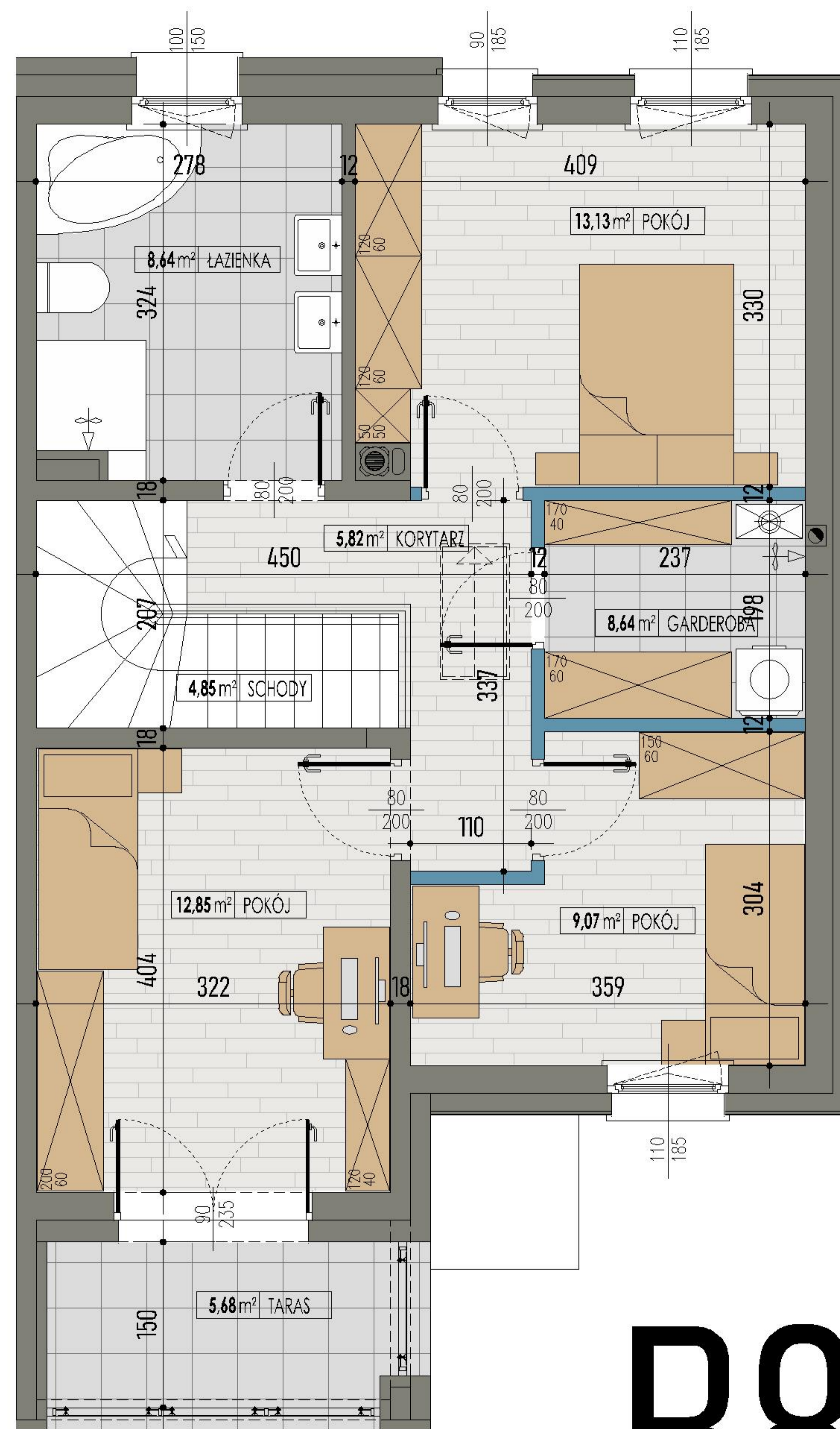
RZUT PIĘTRA
